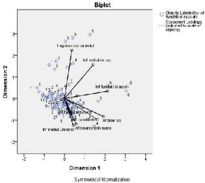
Fig.1. Graficul normalizării simetrice în două dimensiuni, rezultat de programul SPSS 21 prin analiza factorială a componentelor principale
